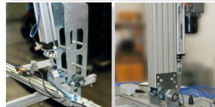
3 Rotazione telaio a ventose con cilindro pneumatico. Sucker frame rotation with pneumatic cylinder
