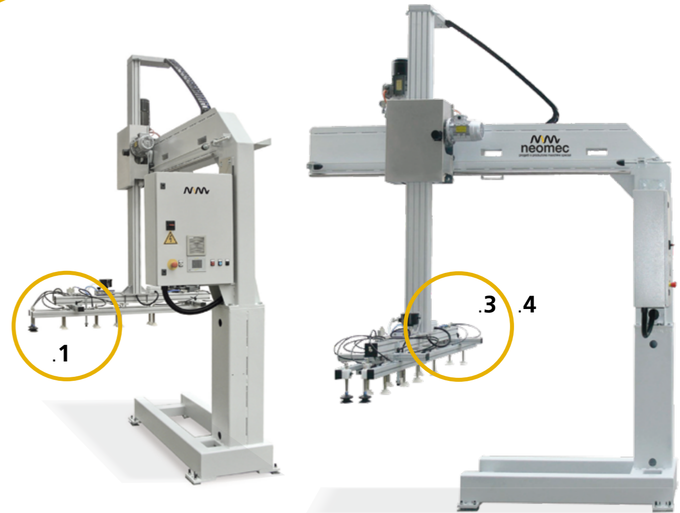
1 Gruppo di presa a ventose per pannelli Sucker gripping unit for panels
