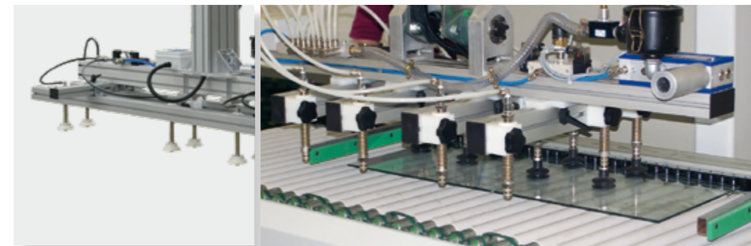
1 Gruppo di presa a ventose per pannelli Sucker gripping unit for panels
