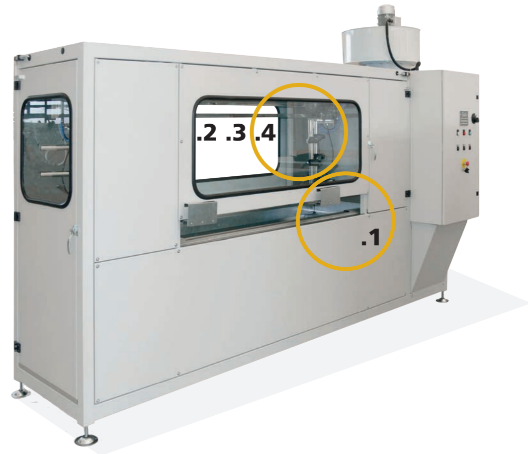
1 Sistema di lettura – ingresso pezzi. Reading system – part entrance.
