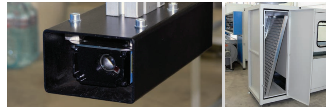
1 Sistema di lettura – ingresso pezzi. Reading system – part entrance.
